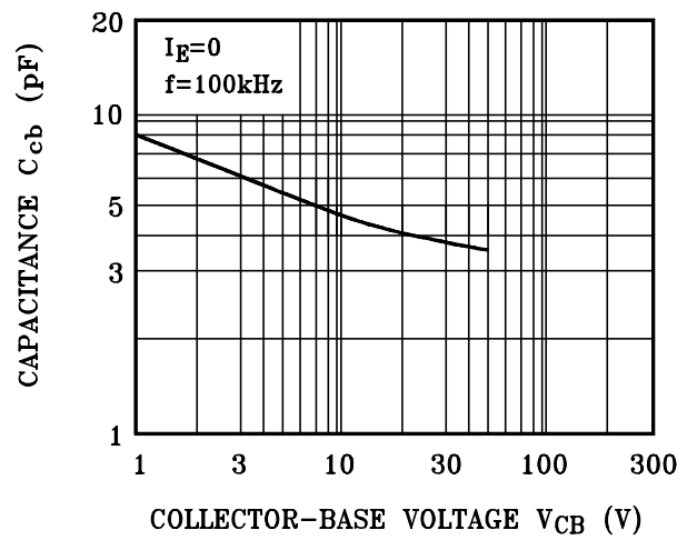
C_{cb} - V_{CB}
