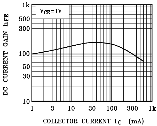
h_{FE} - I_C
