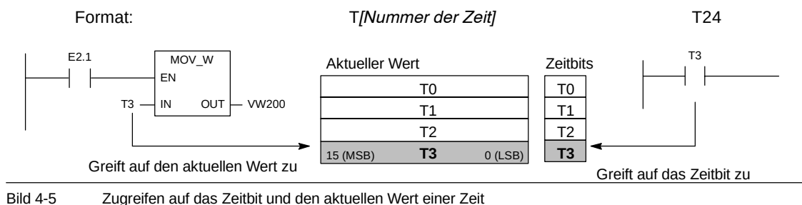
Bild 4-5 Zugreifen auf das Zeitbit und den aktuellen Wert einer Zeit
