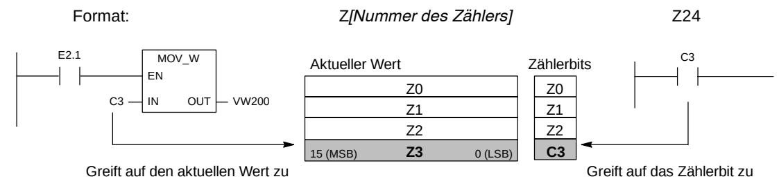
Bild 4-6 Zugreifen auf das Zählerbit und den aktuellen Wert eines Zählers
