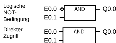
Bild 5-5 FUP-Konventionen
