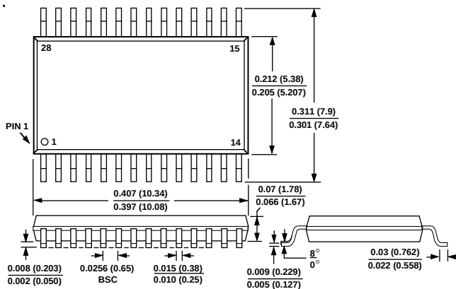
SSOP (RS-28)
