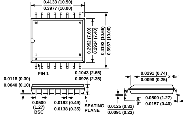
SOIC (R-16)
