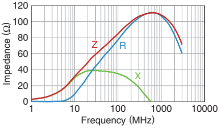
MMZ1608S221A
