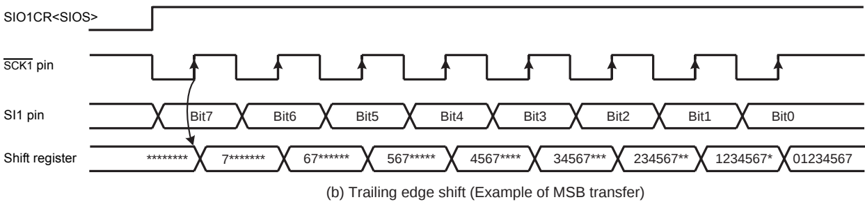
Figure 14-4 Shift Edge
