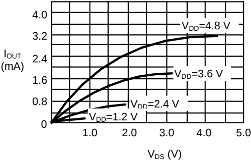
V_{DS} - I_{OUT}
