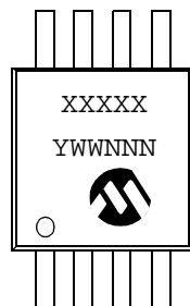
8 引脚 MSOP 封装（固定）
