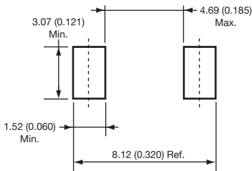
DO-214AB (SMC)
