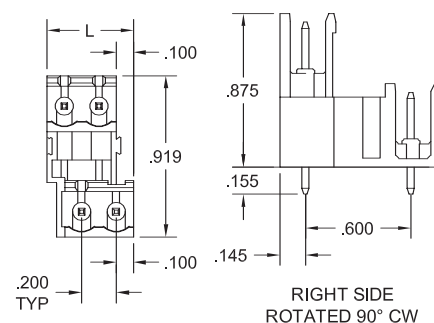
ELFD—Vertical
