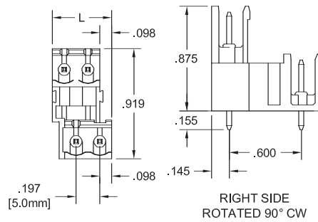
ELFD—Vertical
