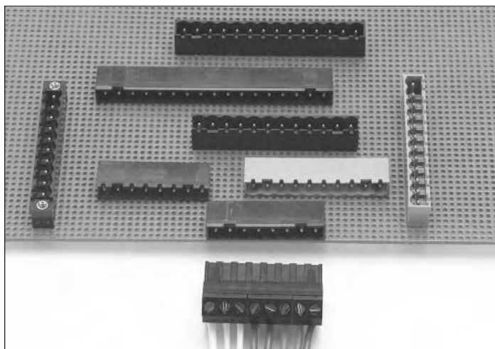
ELFH Horizontal—Eared
