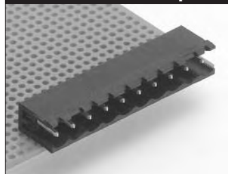
ELFH Horizontal—Open
