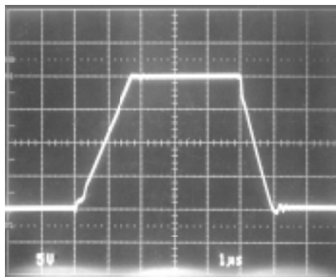
B) LT1057
