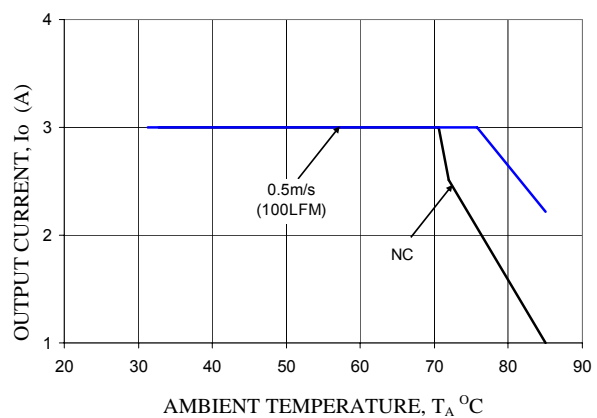
V_o = 5.0V
