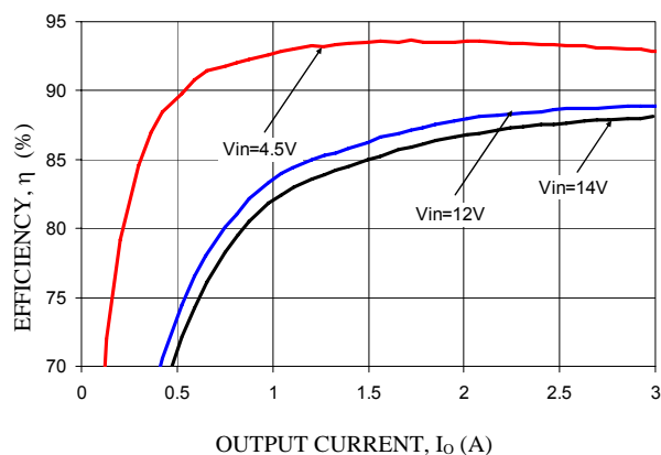
V_o = 2.5V
