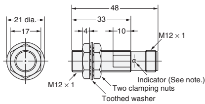
Fig. 20: E2E-X3D□-M1(G) E2E-X2E□-M1/F□-M1
