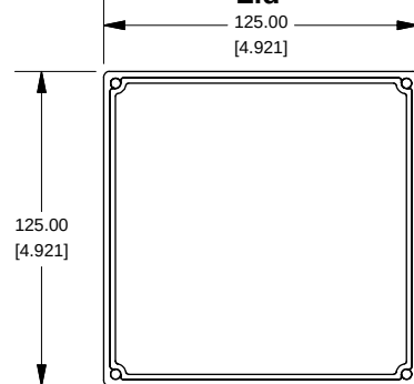
Lid
