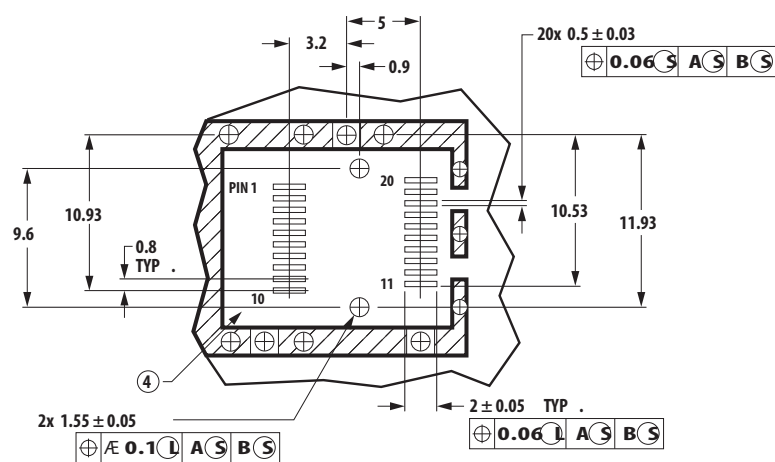
DET AIL 1
