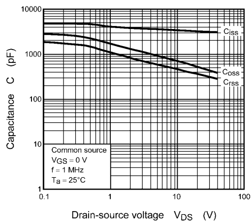
Fig. 9.8 Capacitance - V_{DS}
