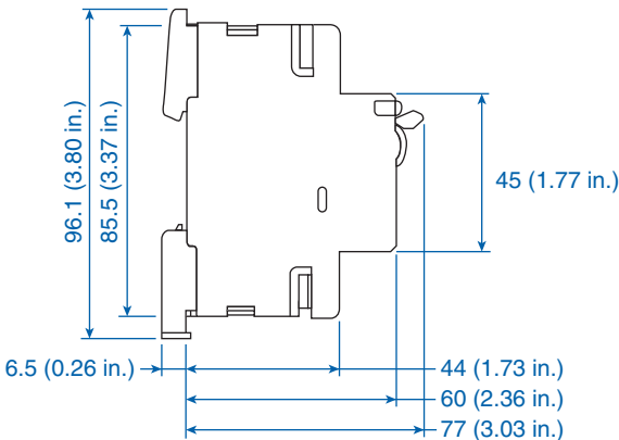
3 POLE
