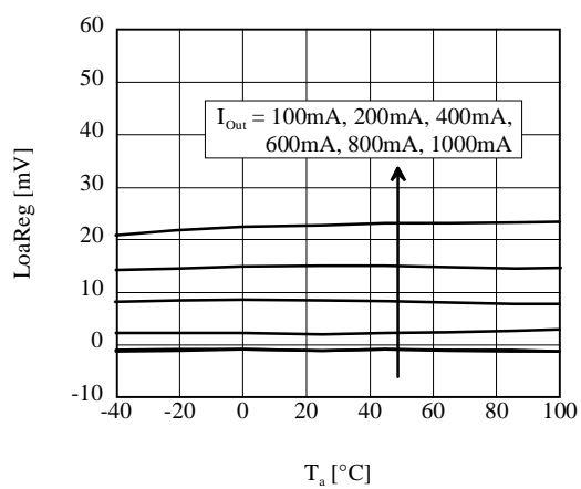
■ LoadReg vs T_a (AP1155ADL)
