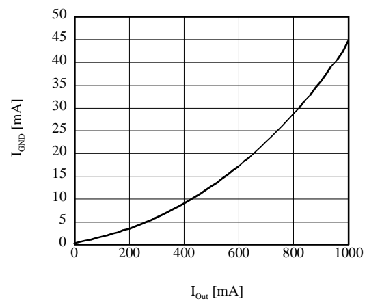
■ I_{\text{GND}} vs I_{\text{Out}} (AP1155ADL)
