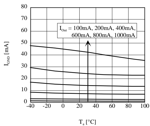
■ I_{\text{GND}} vs T_a (AP1155ADL)
