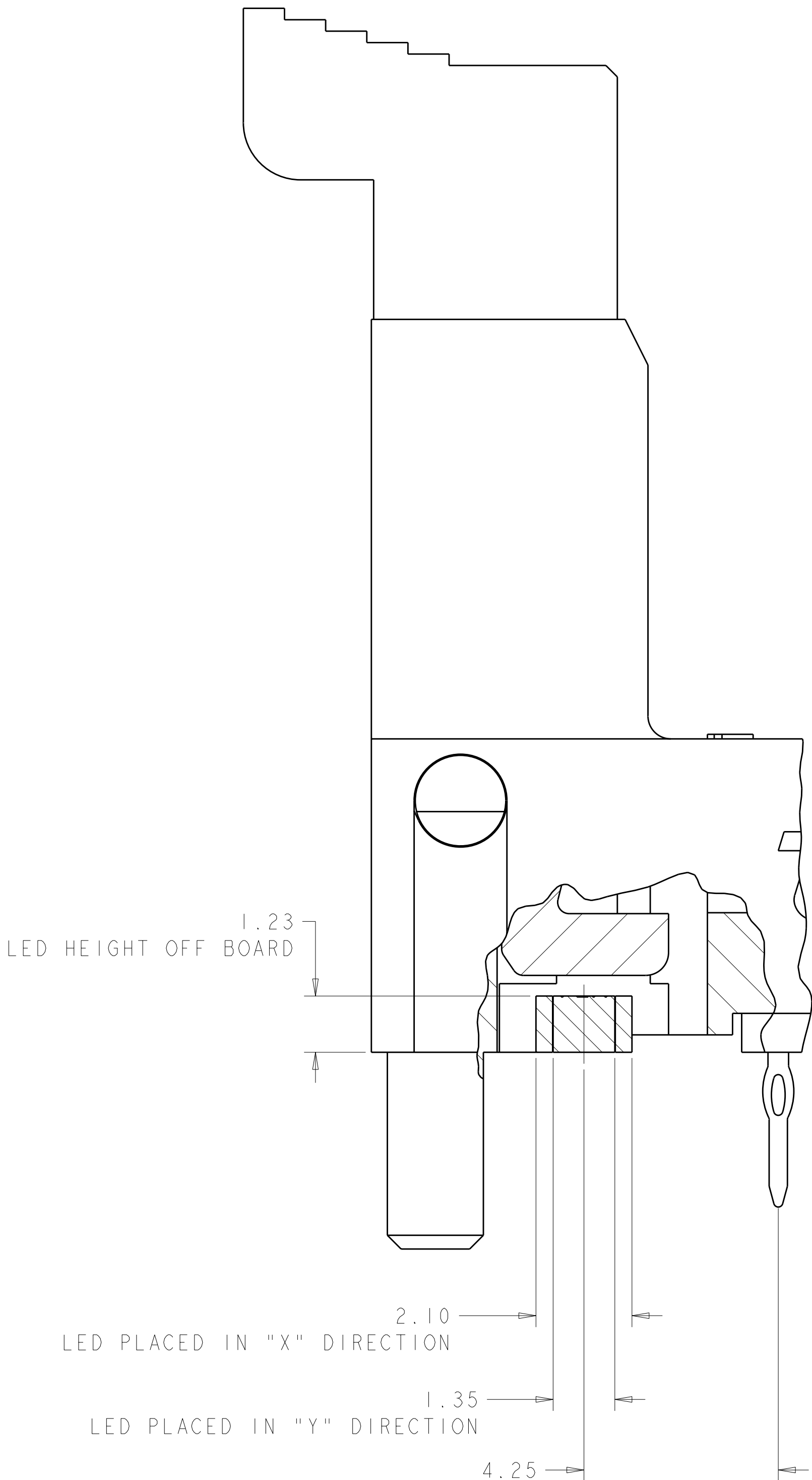
SECTION G-G SCALE 12:1
