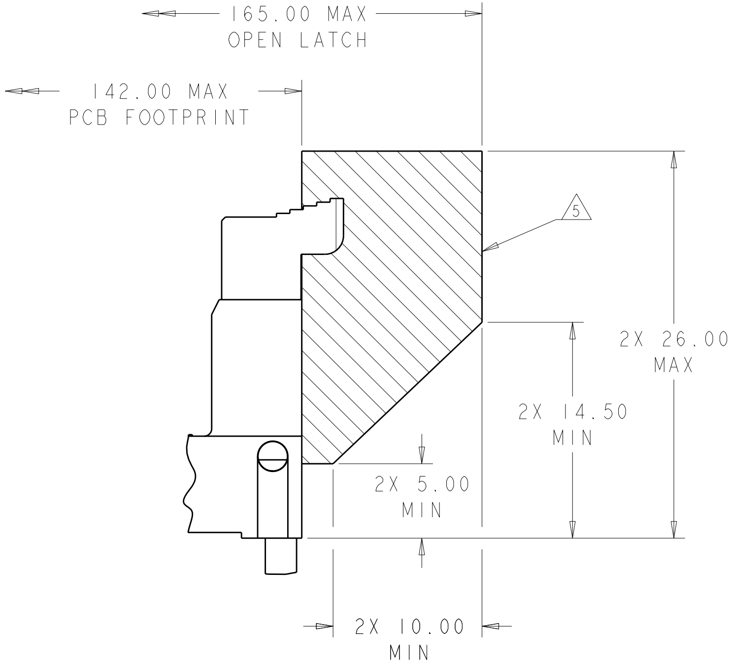
1761623-2 SHOWN
