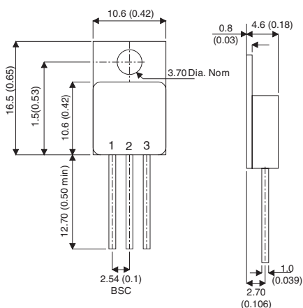
220M-Package (TO-220)
