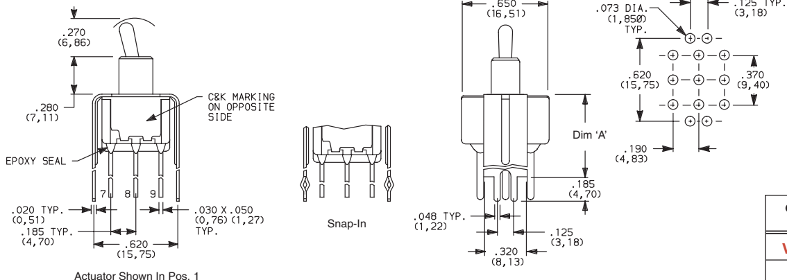
7301MD9__BE 3PDT
