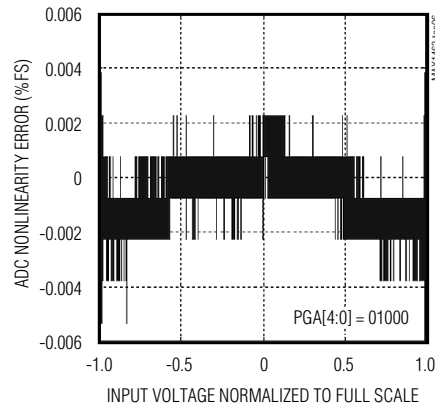
ADC INL
