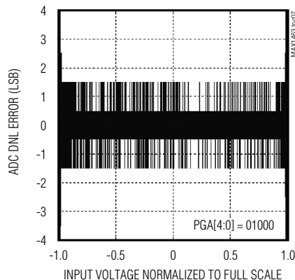
ADC DNL
