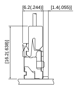
PAF Receptacle + PA Header
