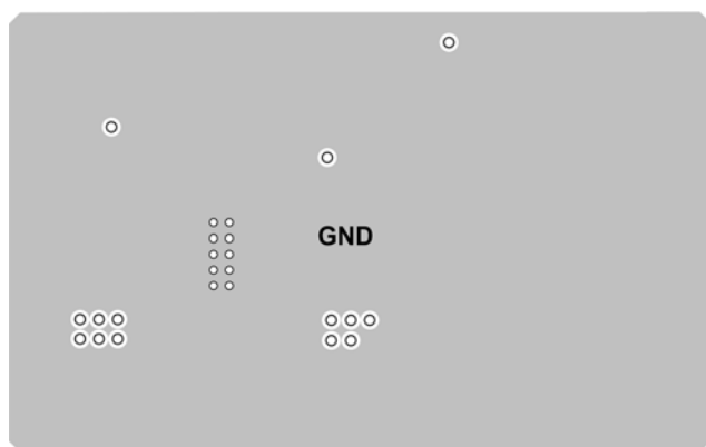
Inner Layer 2
