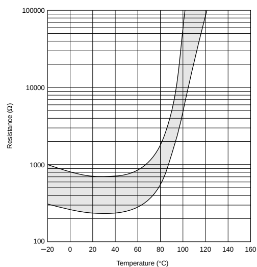
PRF18BD471QS2RB
