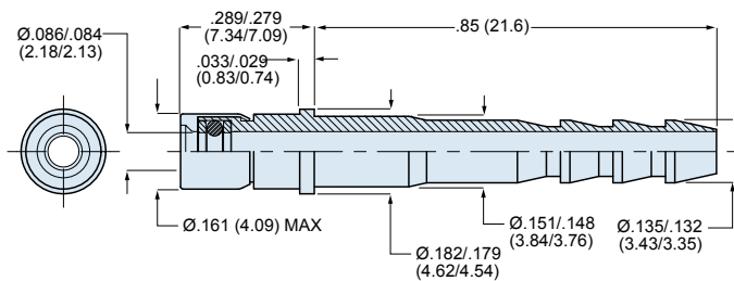
857-010 Socket Contact
