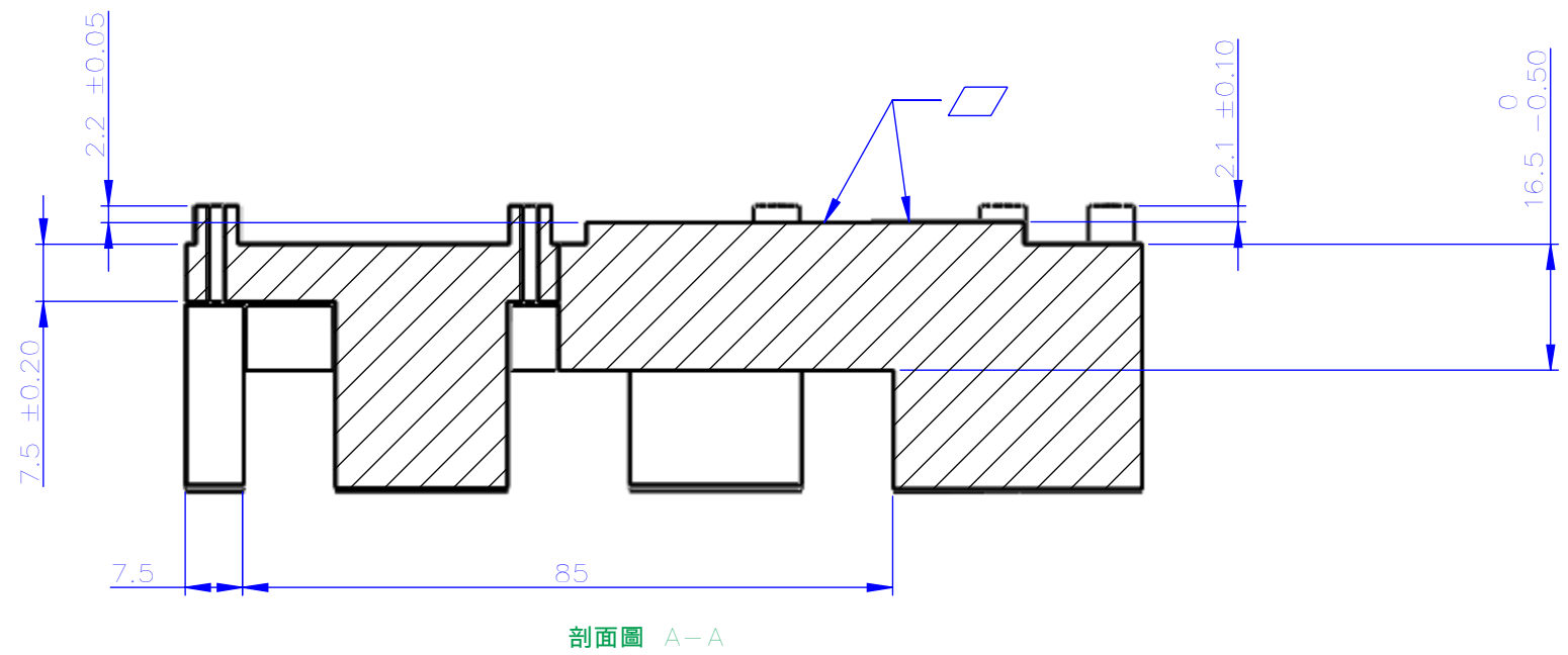
剖面圖 A-A
