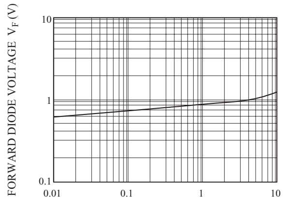
V_F - I_F
