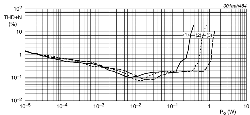
a. G_{V(cl)} = 24 dB
