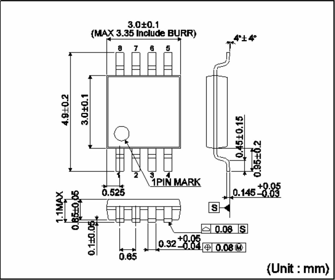
TSSOP-B8J
