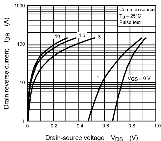
Fig. 8.7 I_{DR} - V_{DS}
