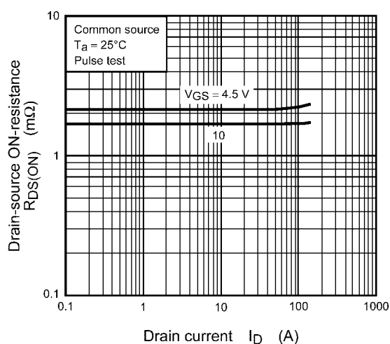
Fig. 8.5 R_{DS(ON)} - I_D
