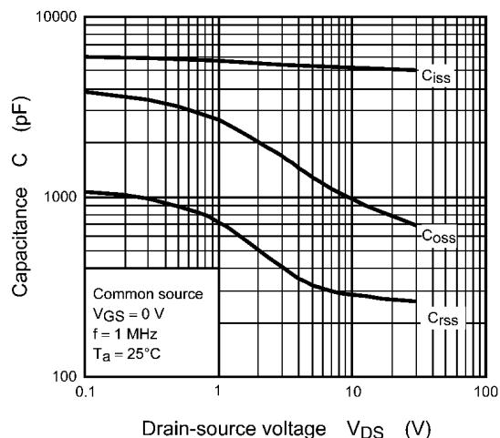
Fig. 8.8 Capacitance - V_{DS}
