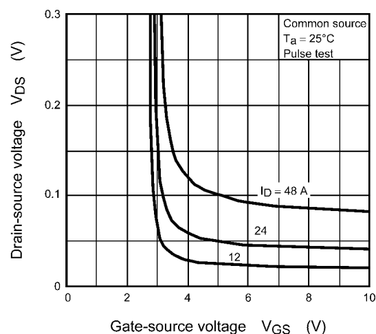
Fig. 8.4 V_{DS} - V_{GS}
