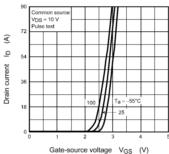
Fig. 8.3 I_D - V_{GS}
