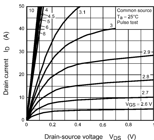
Fig. 8.1 I_D - V_{DS}
