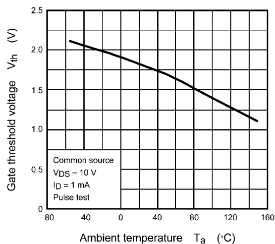
Fig. 8.9 V_{th} - T_a
