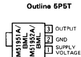
Outline SOT-89
