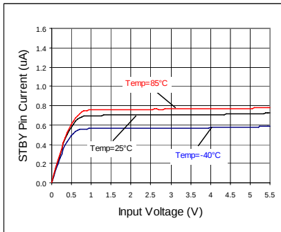
Fig 106. VSTBY - ISTBY
