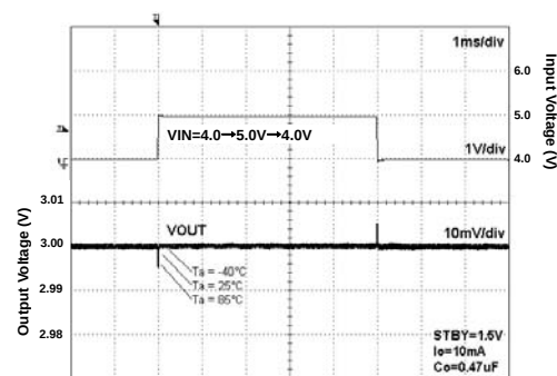
Fig 232. VIN Response
