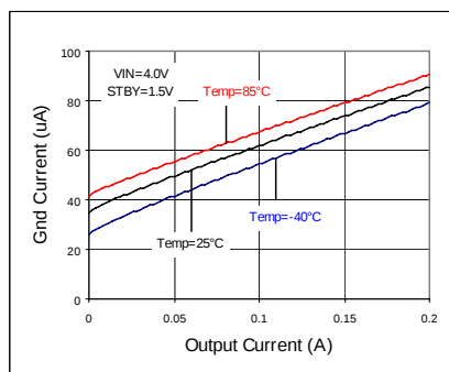
Fig 211. IOOUT - IGND
