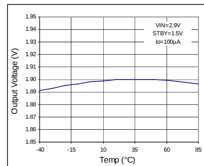
Fig 86. VOUT - Temp
