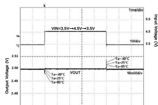
Fig 128. VIN Response
