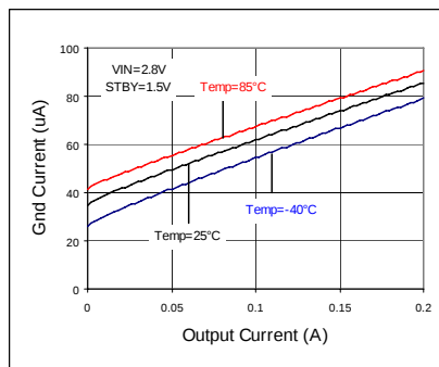
Fig 57. IOUT - IGND
