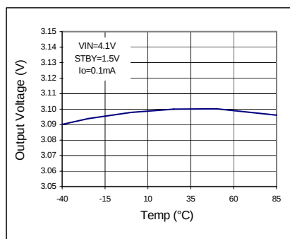
Fig 242. VOUT - Temp
