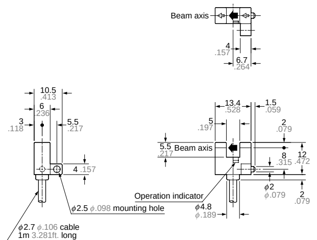
UZJ316 Sensor
