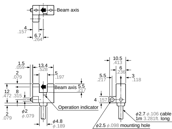
UZZ315 Sensor
