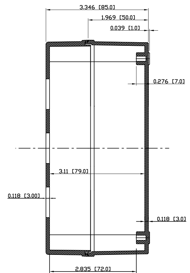
SECTION A-A
