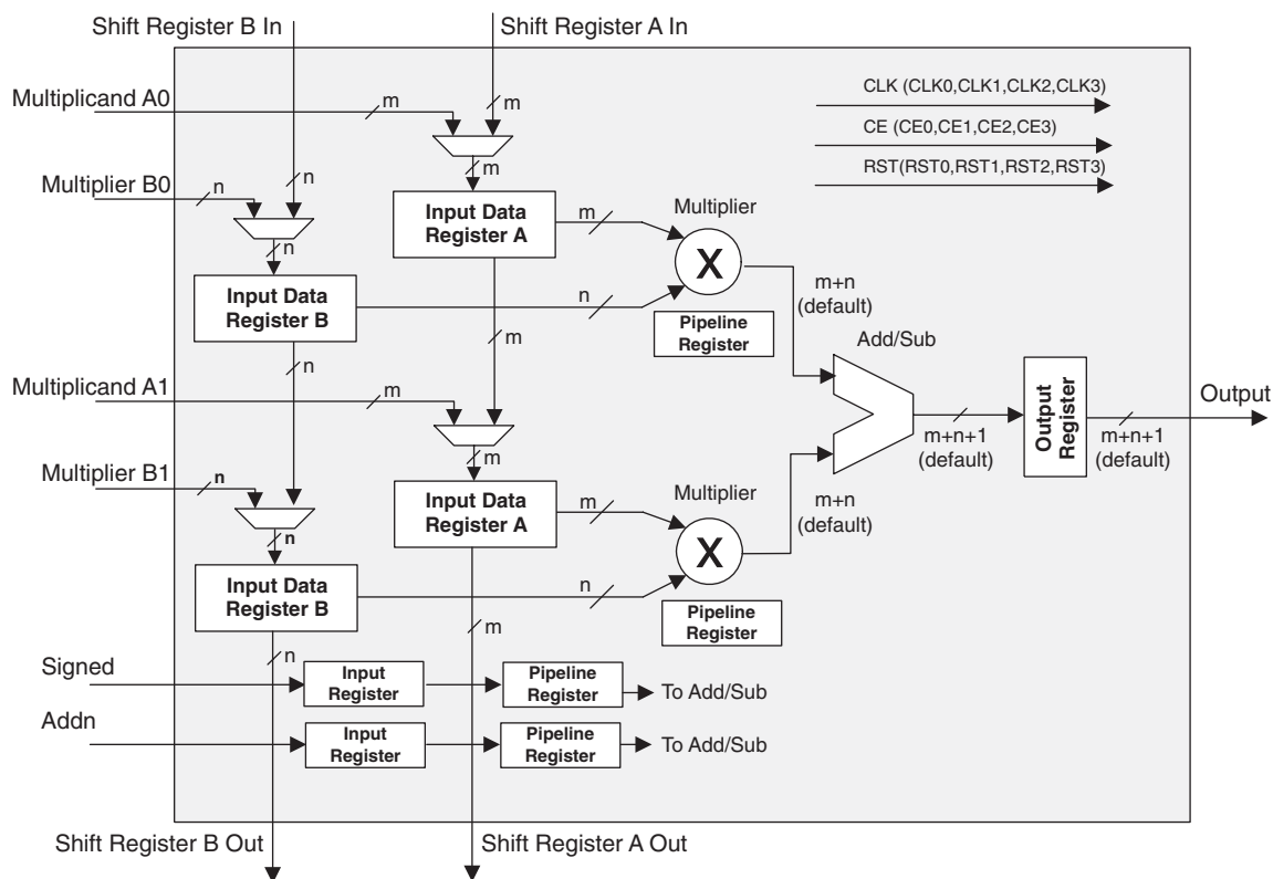
Figure 2-22. MULTADD
