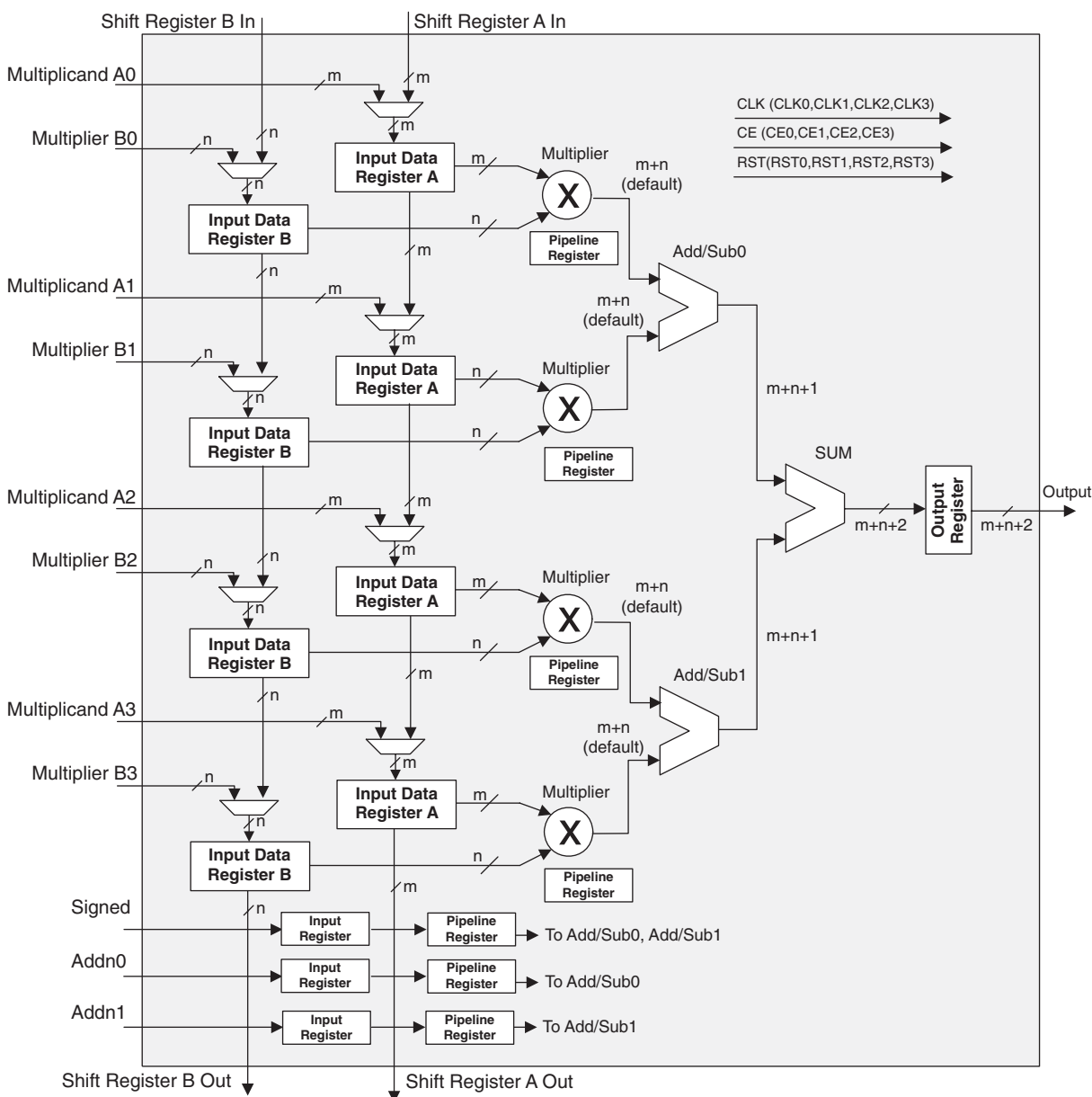
Figure 2-23. MULTADDSUM
