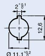
Panel cutout / Durchbruch in Montageplatte
