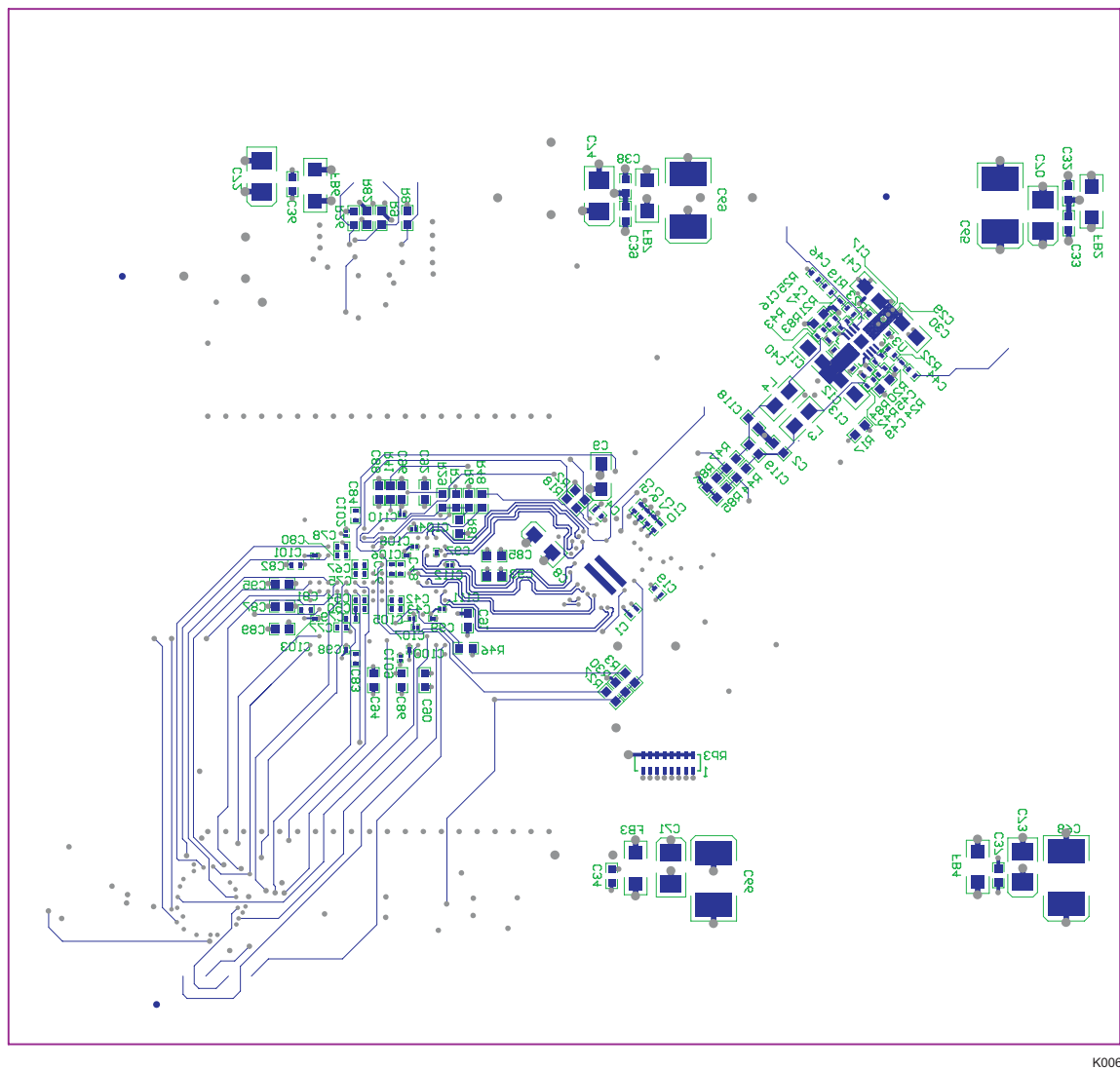
Figure 9. Layer 6, Bottom Layer
