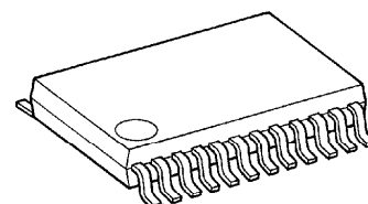
SSOP24-P-300-0.65A
