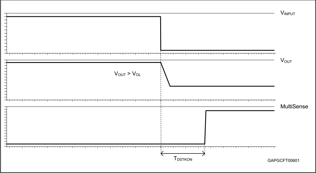
Figure 9. T_{DSTKON}
