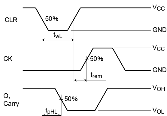
図4 クリアモード (TC74VHC161)
