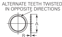
Lockwasher
