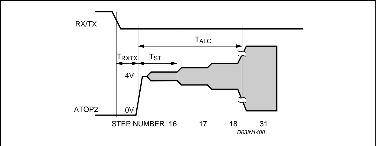
Figure 16. PLI Startup Timing Diagram
