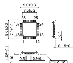
VQFP48
