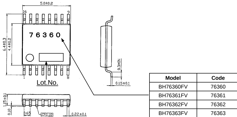
SSOP-B16 (unit: mm)
