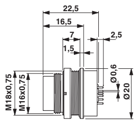
Einlötlanschluss: PV..P1N22HG00
