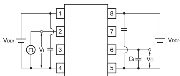
Fig. 9 t_{PHL}/t_{PLH}
