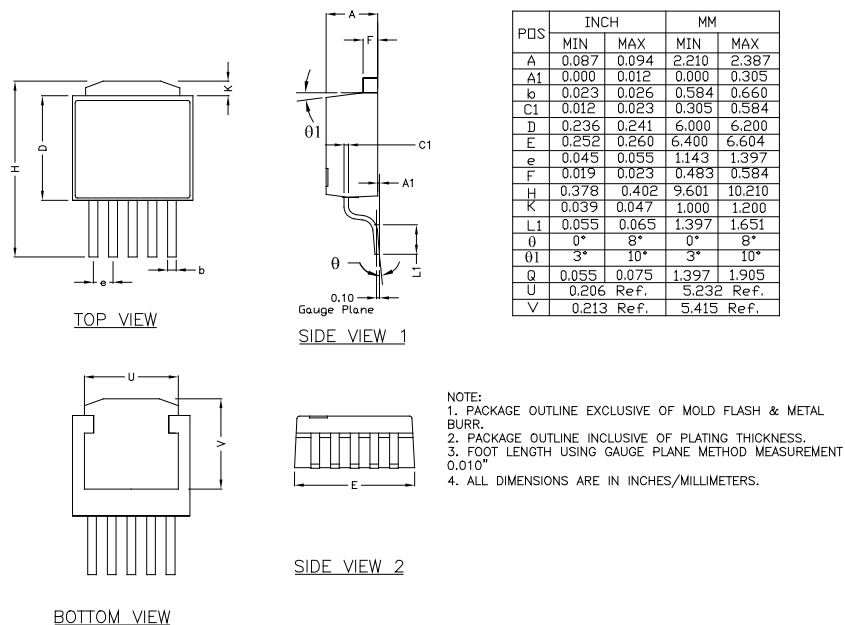
5-Pin TO-252 (D)
