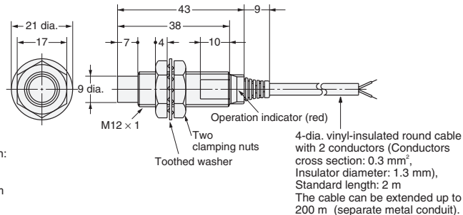
Fig. 12: E2E-X5MY
