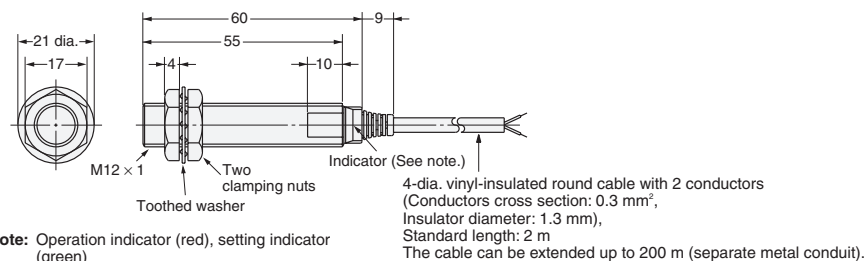
Fig. 13: E2E-X3T1
