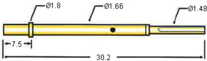
Dimensions : Millimetres
