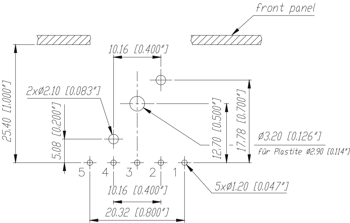
Print-Bohrplan (Bestückungsseite)
